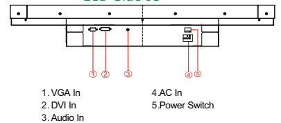
LCD Side IO
